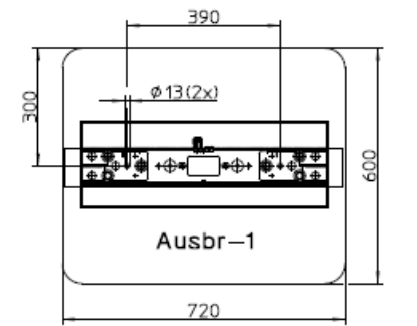
Lochbild für optionale Bodenverschraubung
