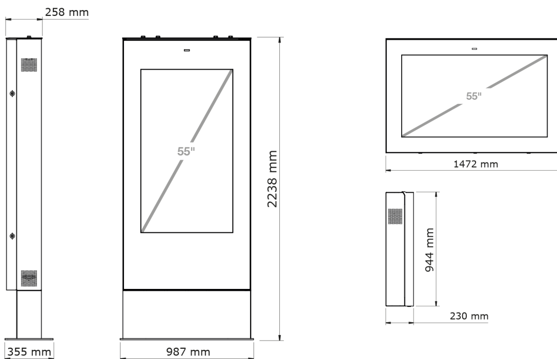
SELKET 55"
